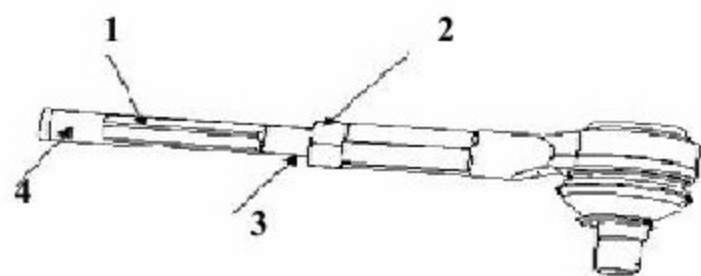
1. 转向横拉杆 3. 转向横拉杆端头 2. 紧固螺母 4. 作标记处
